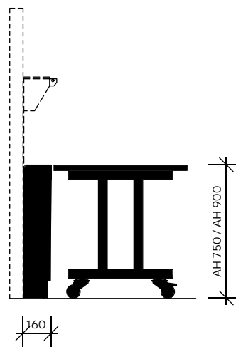
Vorsatzgestell mit fahrbarem Anstellstisch
